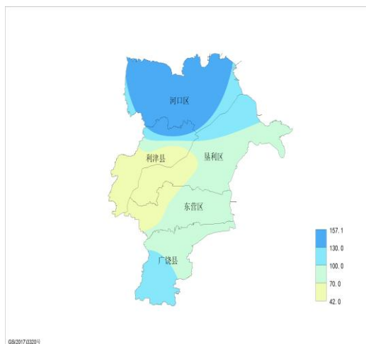
东营市 7 月下旬降水量分布图
