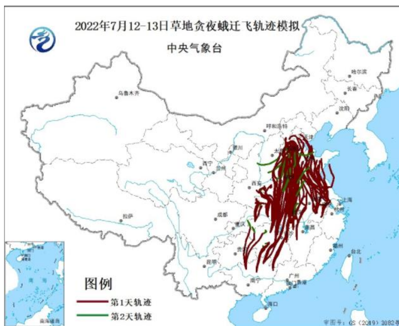
7月12~13日草地贪夜蛾迁飞轨迹模拟
