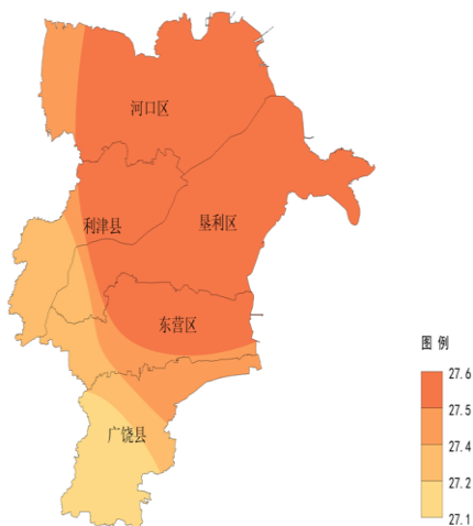
东营市 7 月份平均气温分布图
