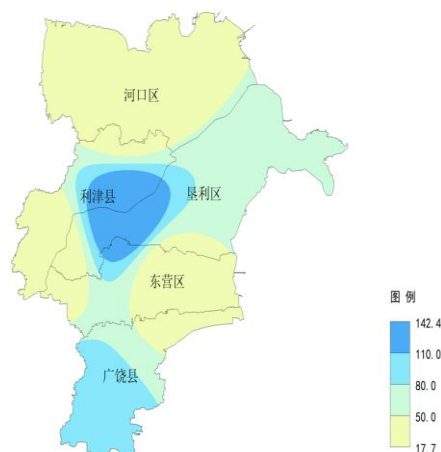
东营市 7 月下旬降水量分布图
