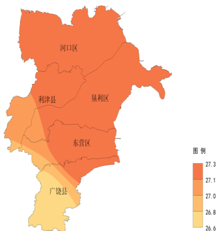
东营市 7 月下旬平均气温分布图
