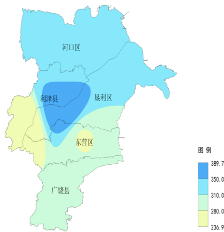
东营市 7 月份降水量分布图
